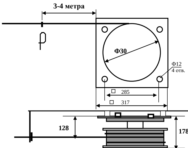
Установка ДВ-22
