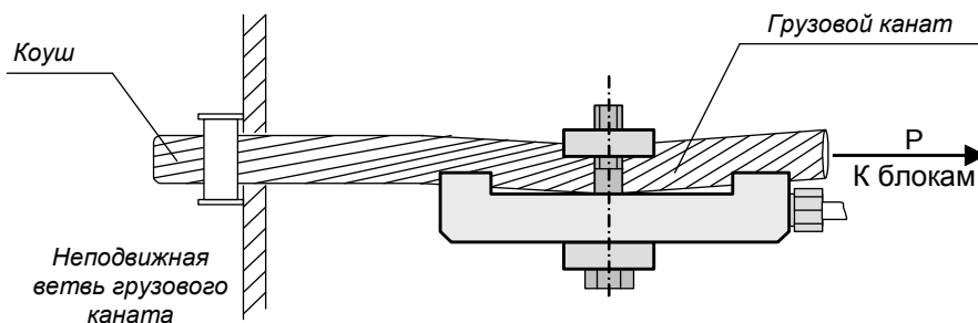
Рисунок 8 – Установка ДУКЦ
