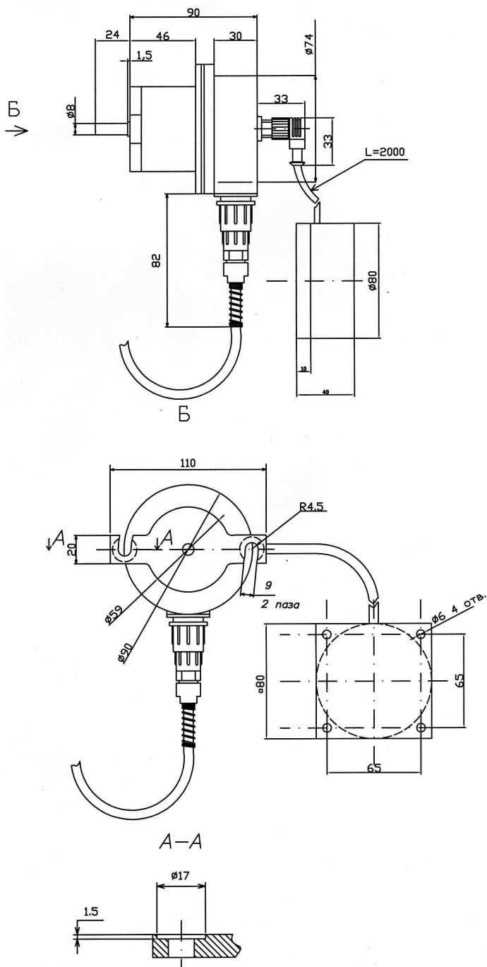
Рисунок 5 – Габаритные и присоединительные размеры датчика ДПИ
