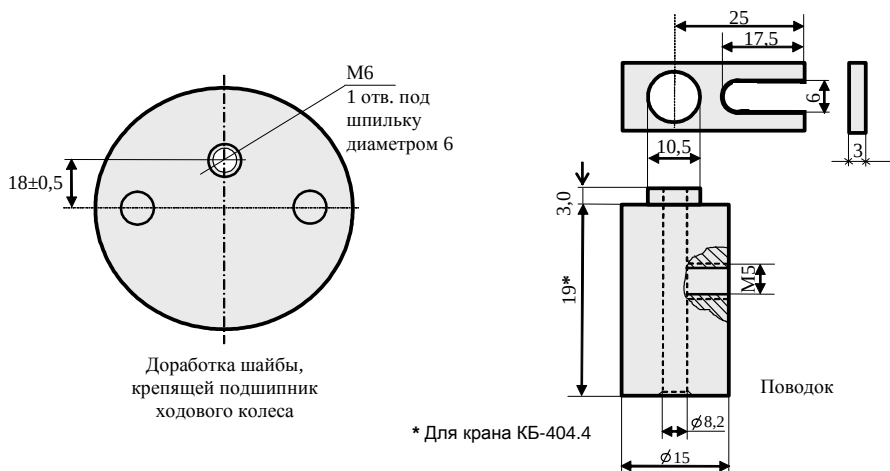
Рисунок 8 – Пример изготовления поводка для датчиков пути и вылета
