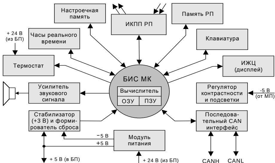
Рисунок 8 - Блок-схема БОИ
