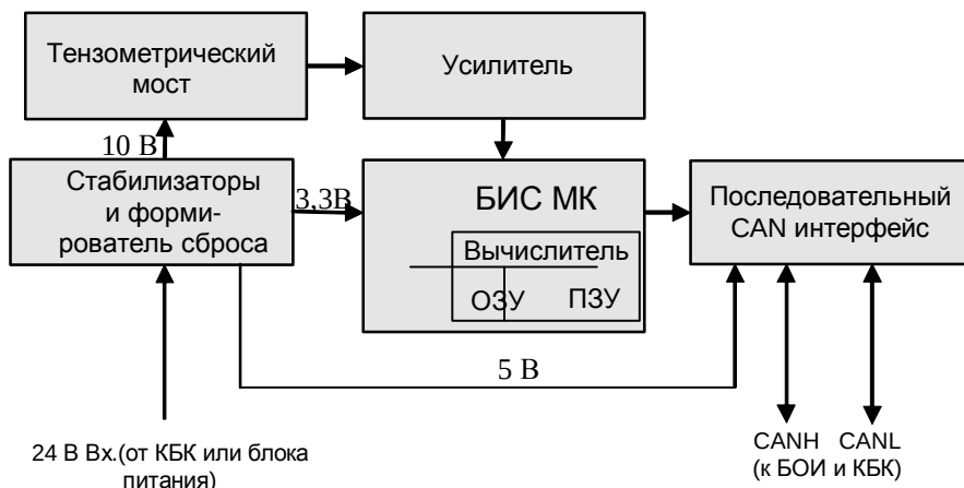
Рисунок 13 - Блок-схема ДУЦ
