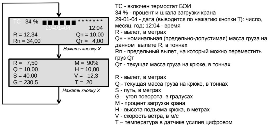
сунок 31 - Вид информационных окон БОИ
