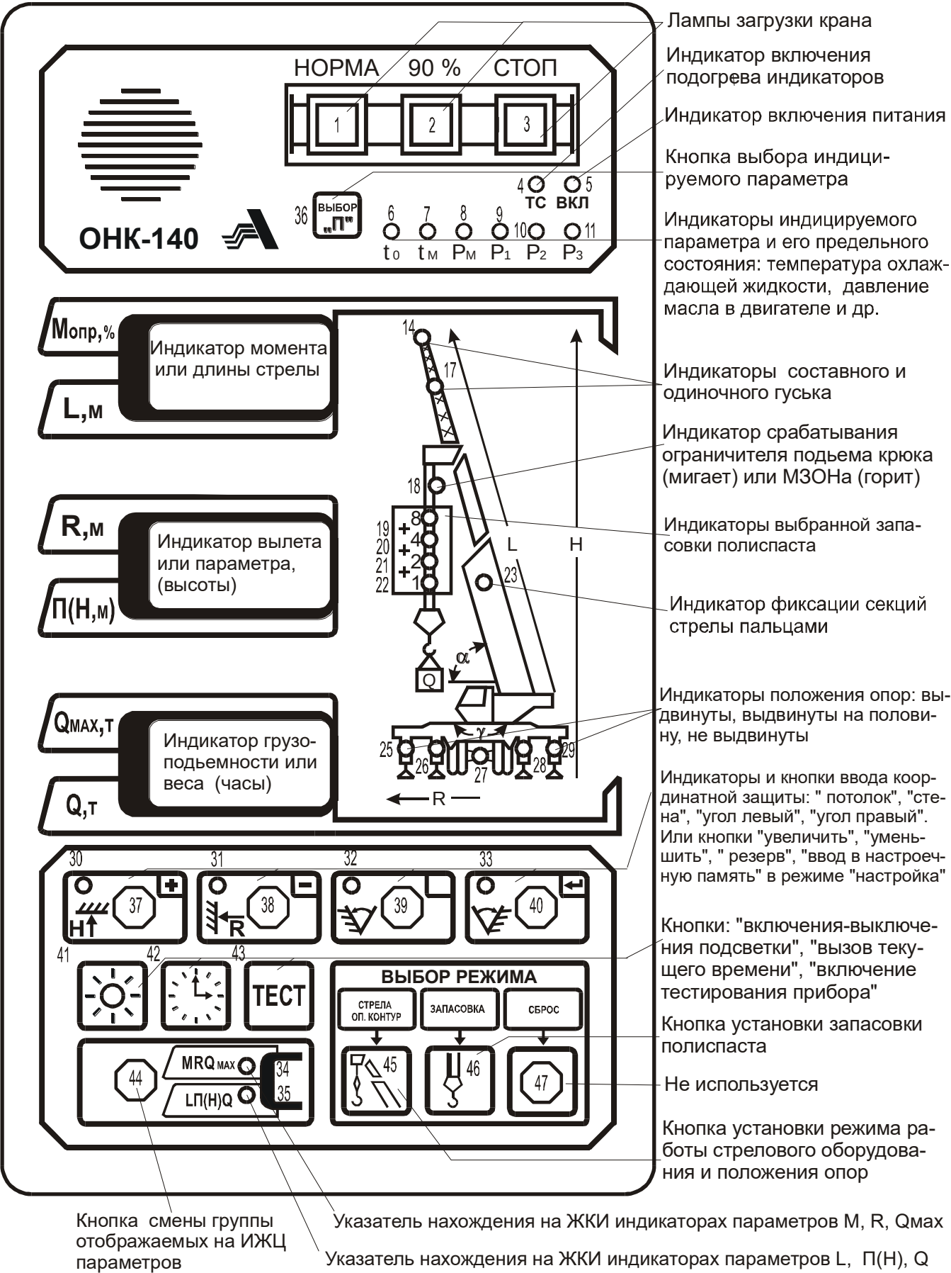
Рисунок 2 - Лицевая панель БОДа
