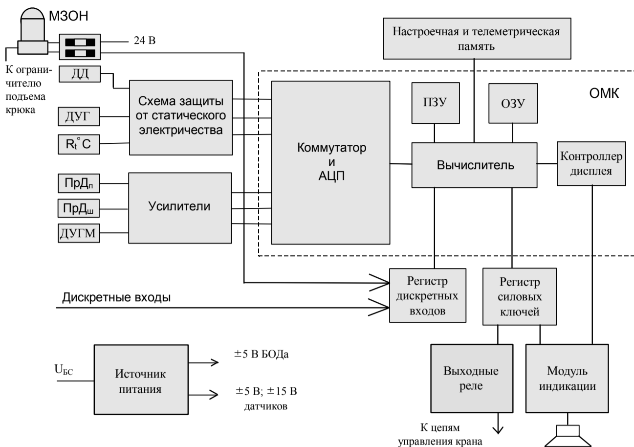
Рисунок 1- Блок-схема ограничителя
